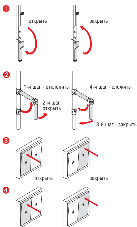
Запертое положение
